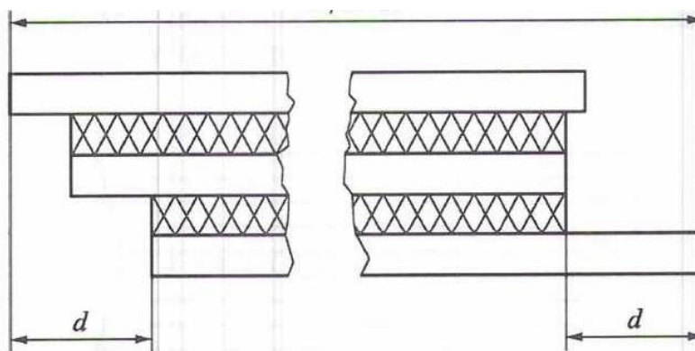
Obrázok č. 5 max. posunutie u vrstvených skiel ( presah skla d)
