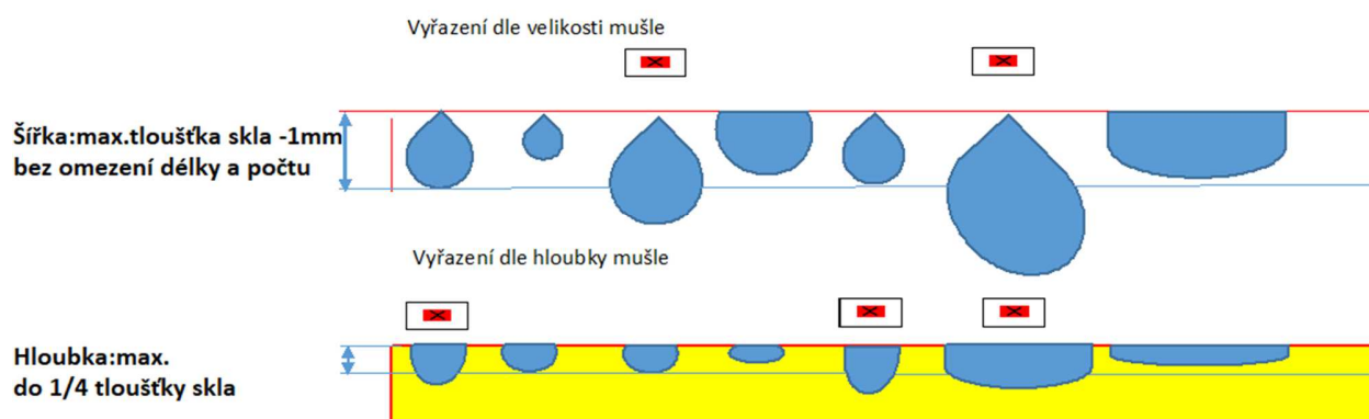
Obrázok 3 – Posudzovanie chýb hrán podľa veľkosti a hĺbky mušle.
